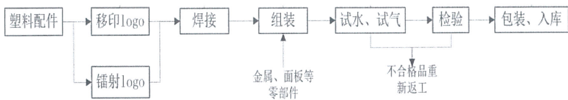
图2-1 金属卫浴制品生产工艺流程图
